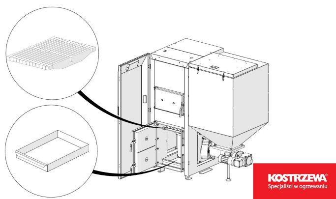
Рис. 2 Колосники для дров, ящик для золы
